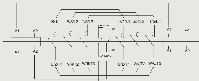
Типова комутаційна схема реверсивного контактора
